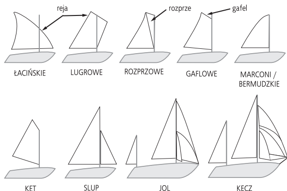
Rysunek 1. Rodzaje ozaglowania i typy ozaglowania
