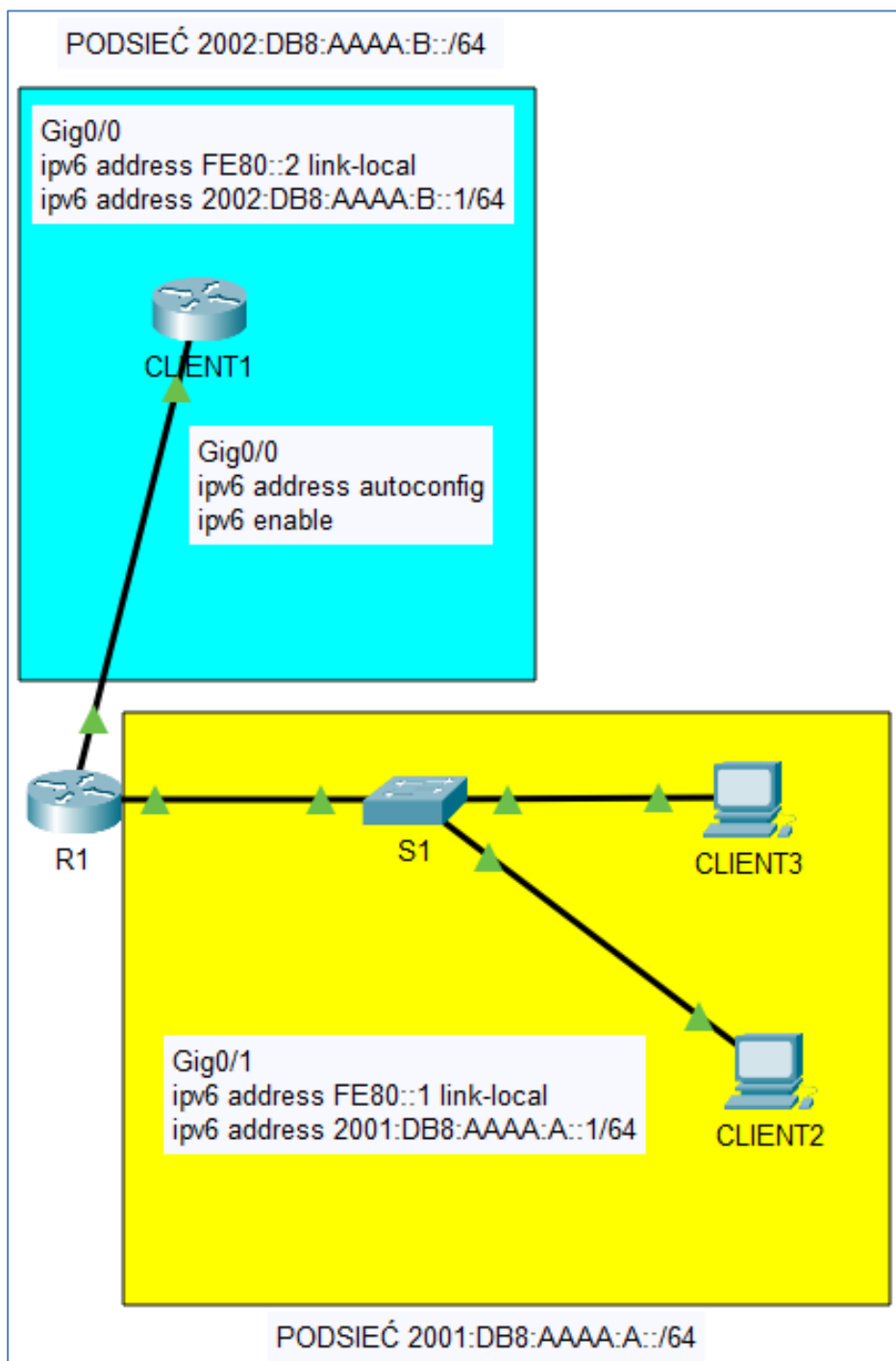
Rysunek 3.15 Topologia sieci IVP6 z metodą SLAAC
