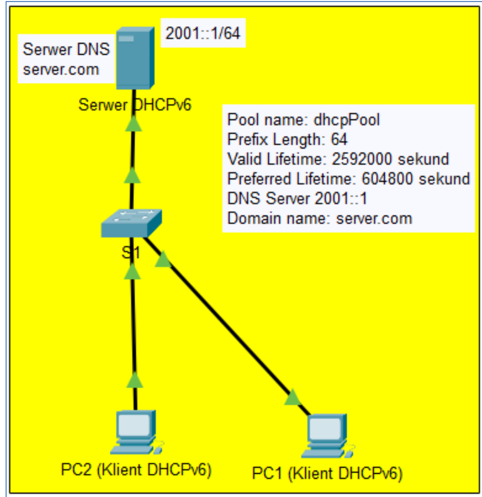
Rysunek 3.31 Topologia sieci IPV6 /64 z serwerem DHCPv6
