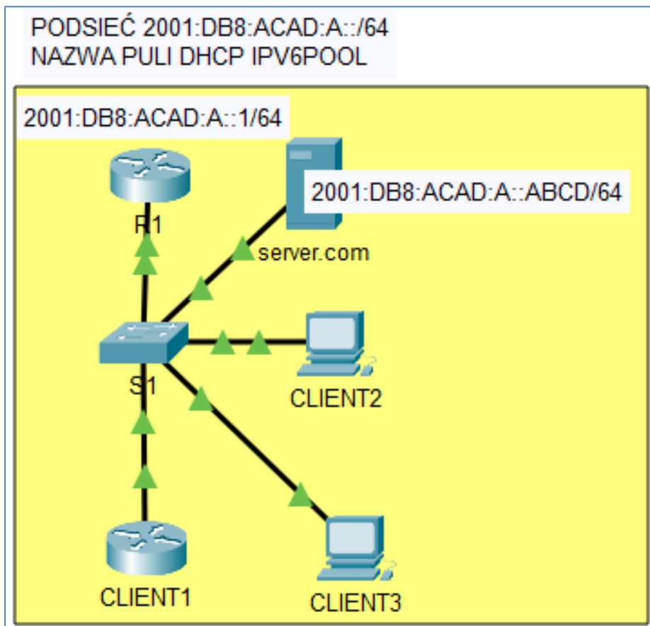
Rysunek 3.19 Topologia sieci IPV6 z metodą SLAAC i bezstanowym DHCPv6
