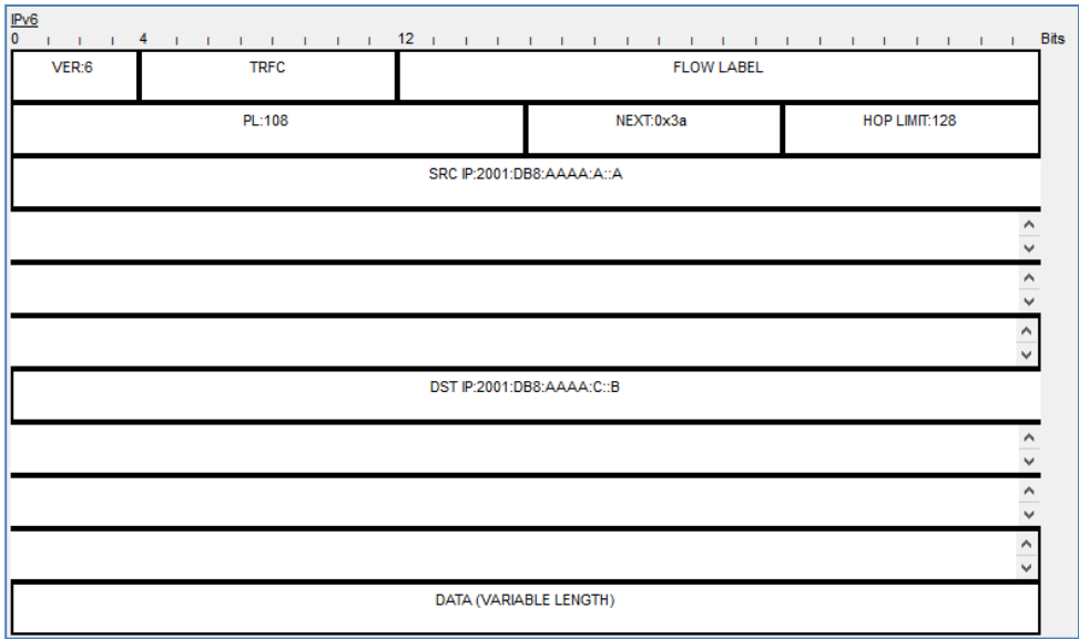
Rysunek 3.2. Przykładowy pakiet IPV6 w programie Packet Tracer
