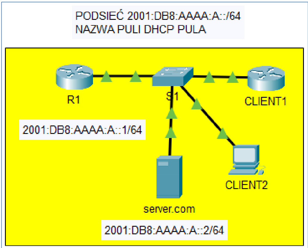
Rysunek 3.26 Topologia sieci IPV6 ze stanowym DHCPv6
