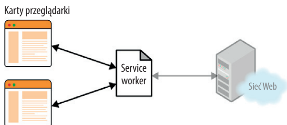
Rysunek 1-4 Strony komunikujące się ze skryptem service worker, gdy użytkownik jest w trybie offline
